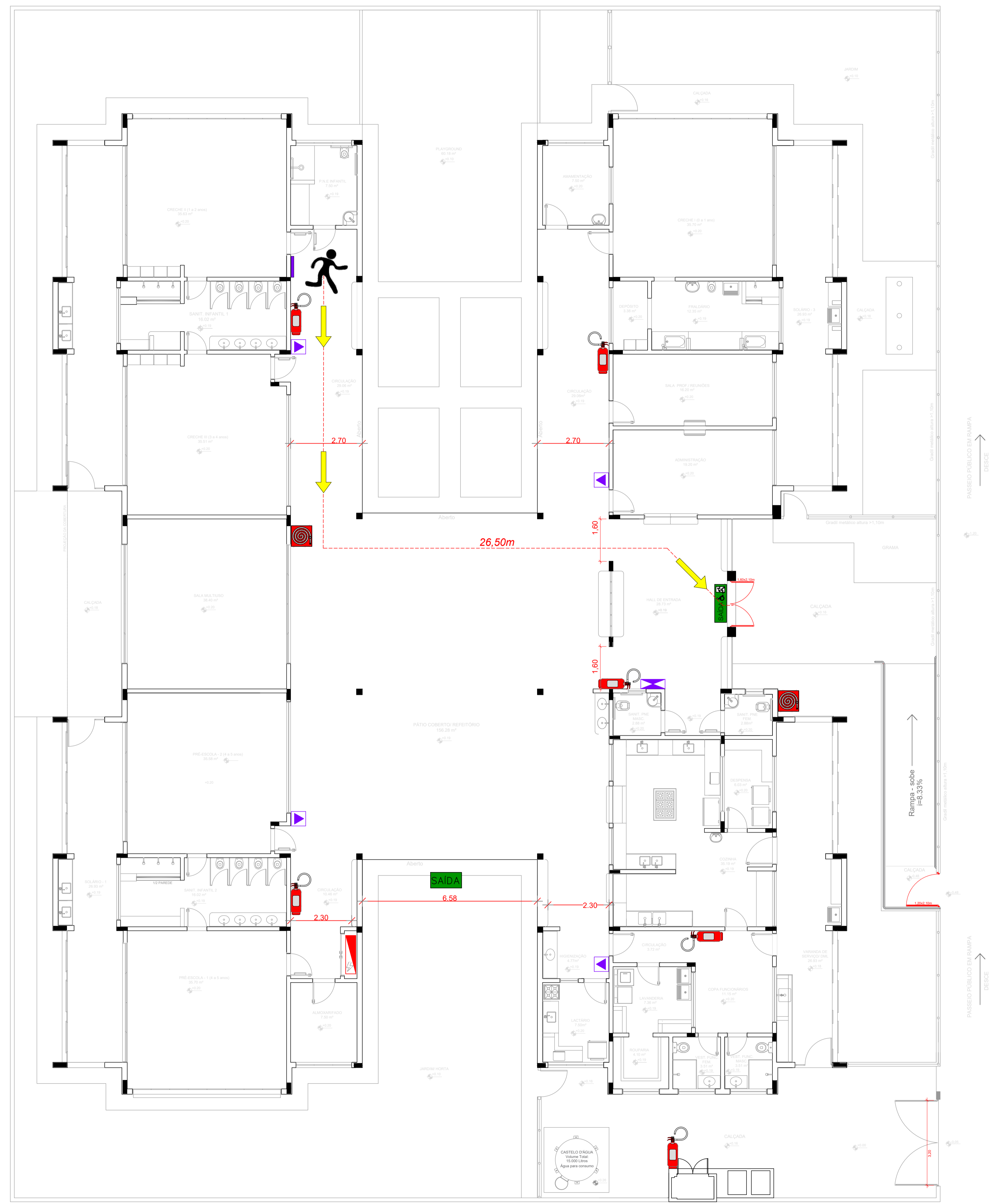
1 PLANTA DE EMERGÊNCIA - ROTAS DE FUGA SEM ESCALA
