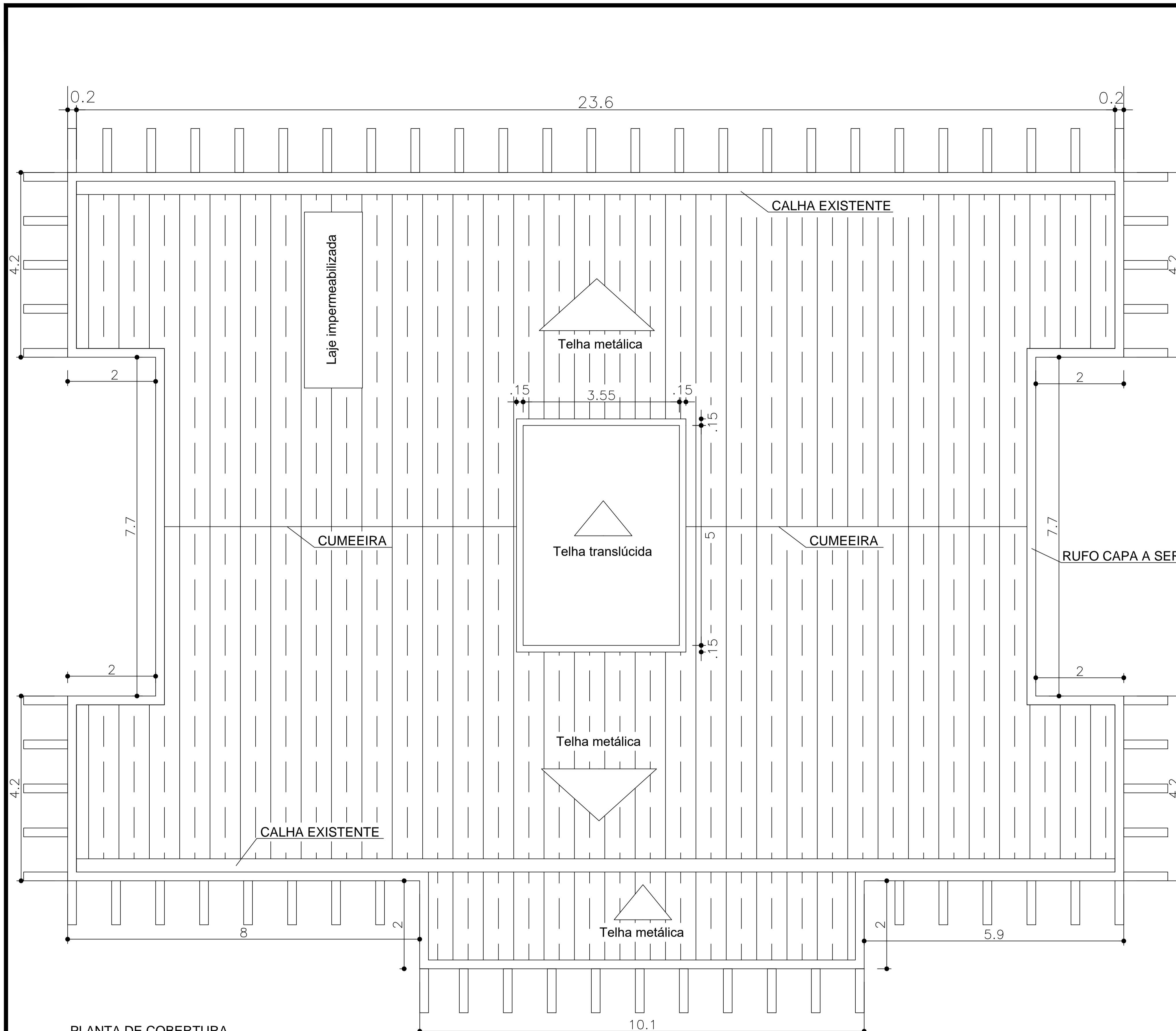
PLANTA DE COBERTURA ÁREA: 375,80m 2 Esc: 1/100
