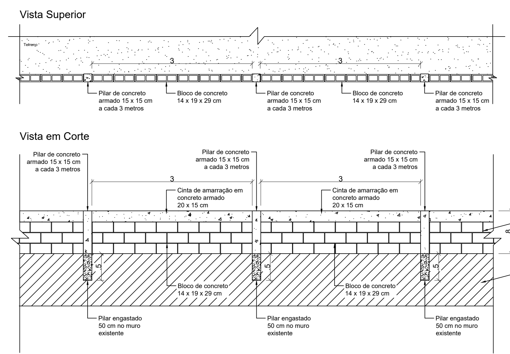
Detalhe Genérico Muro Esc: 1/50
