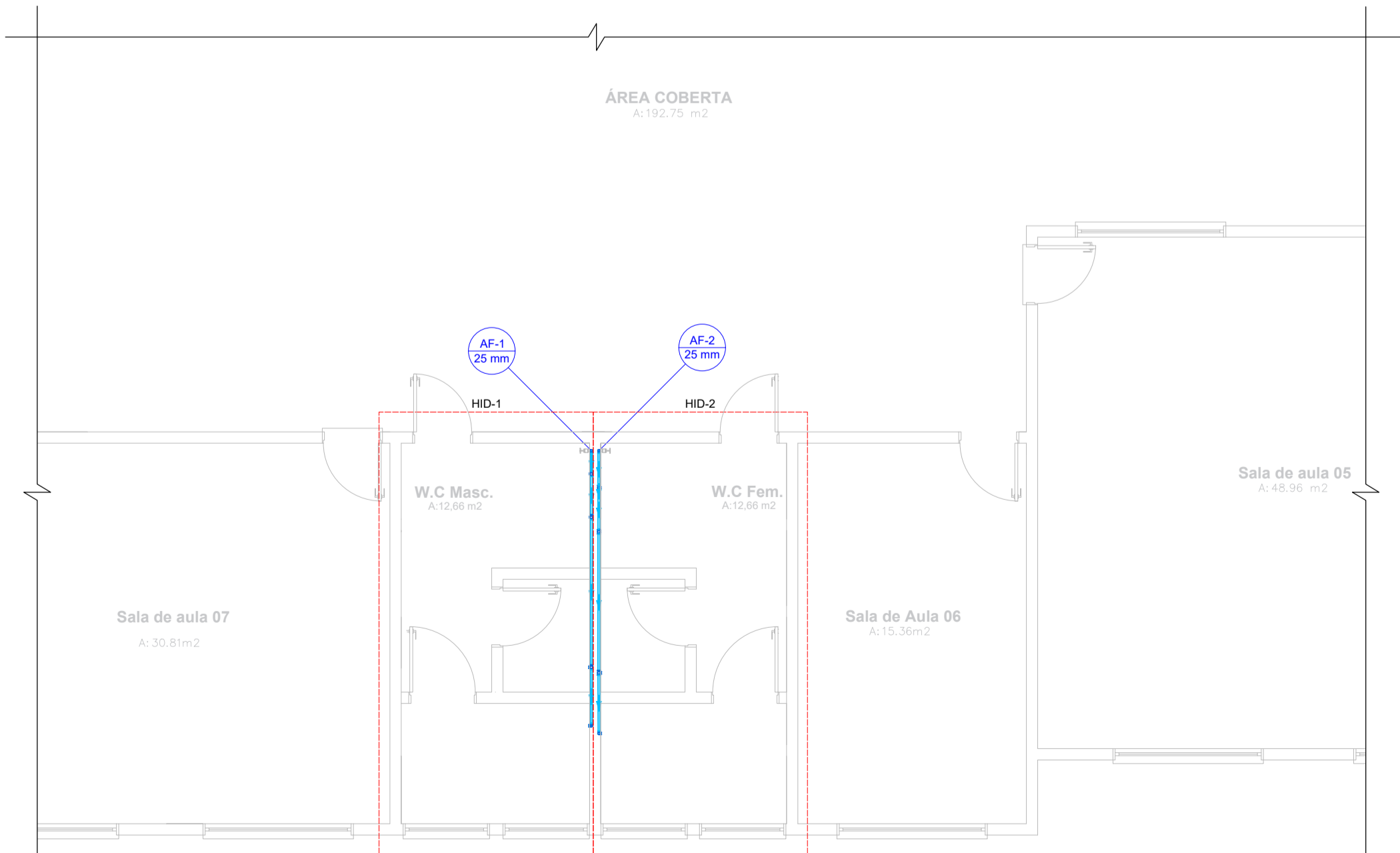
Planta Baixa Hidráulico Escala 1:50
