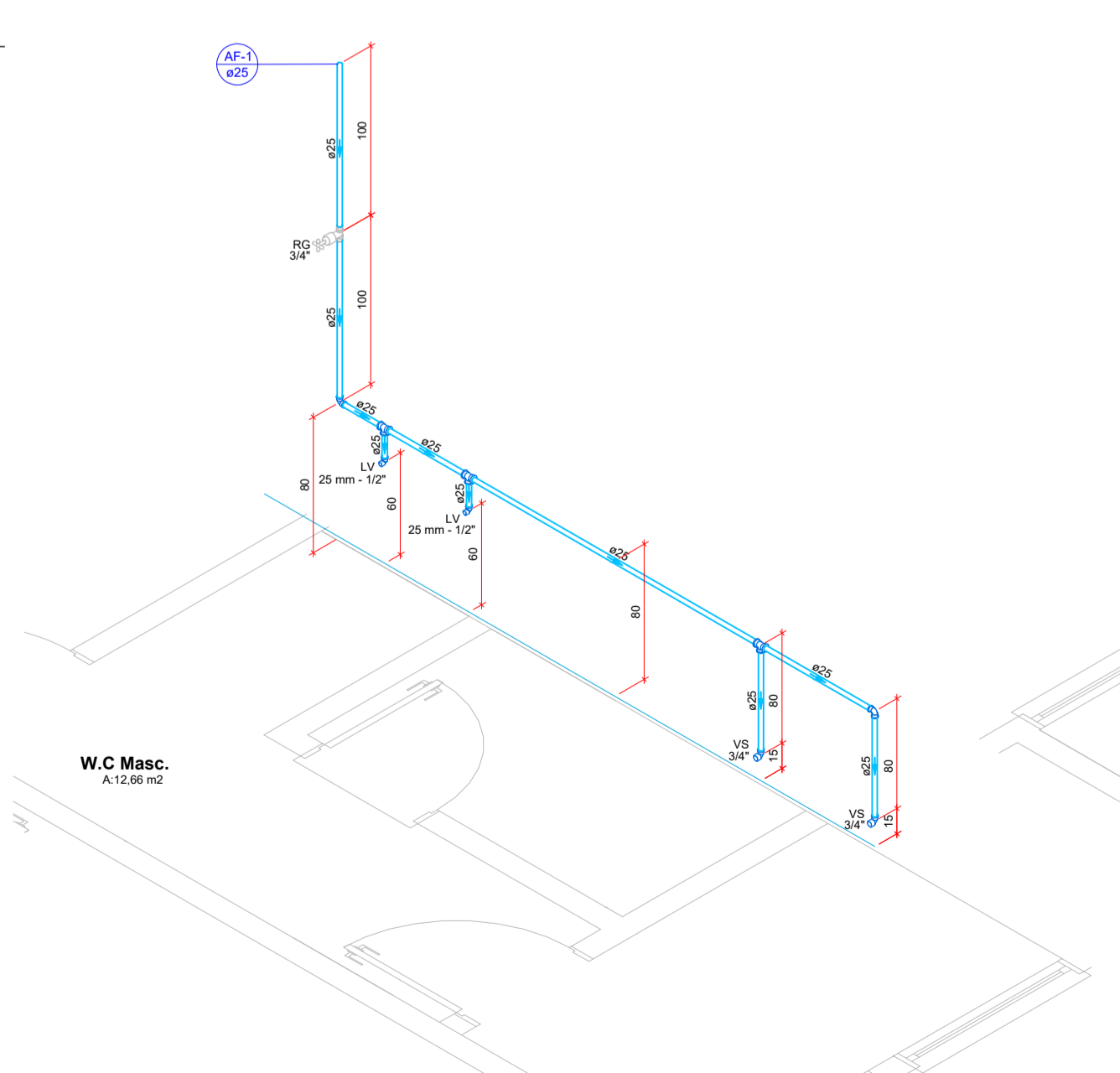
Detalhe HID-1 Escala 1:25
