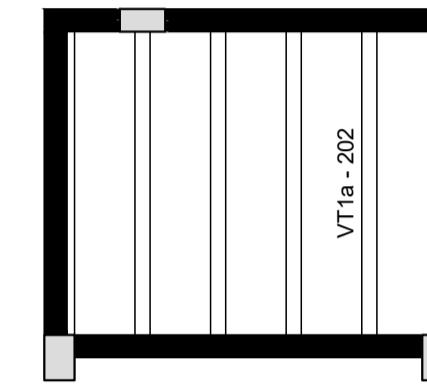
Planta de vigotas pré-moldadas escala 1:50
