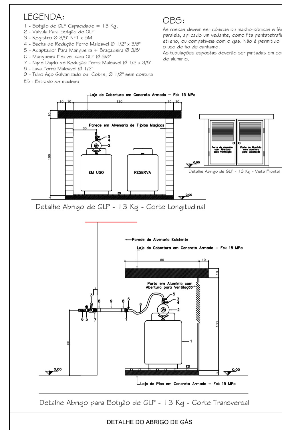
DETALHAMENTO ABRIGO DE GÁS Sem Escala
