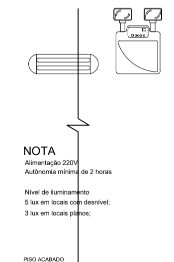
DETALHAMENTO ILUMINAÇÃO DE EMERGÊNCIA Sem Escala
