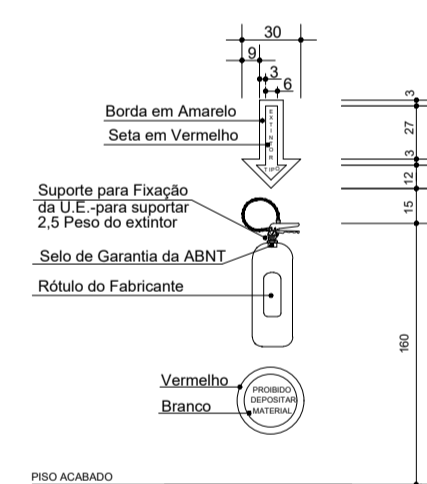
DETALHAMENTO EXTINTORES Sem Escala
