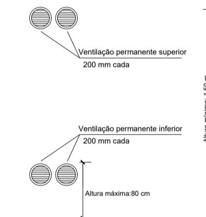
DETALHAMENTO VENTILAÇÃO PERMANENTE Sem Escala
