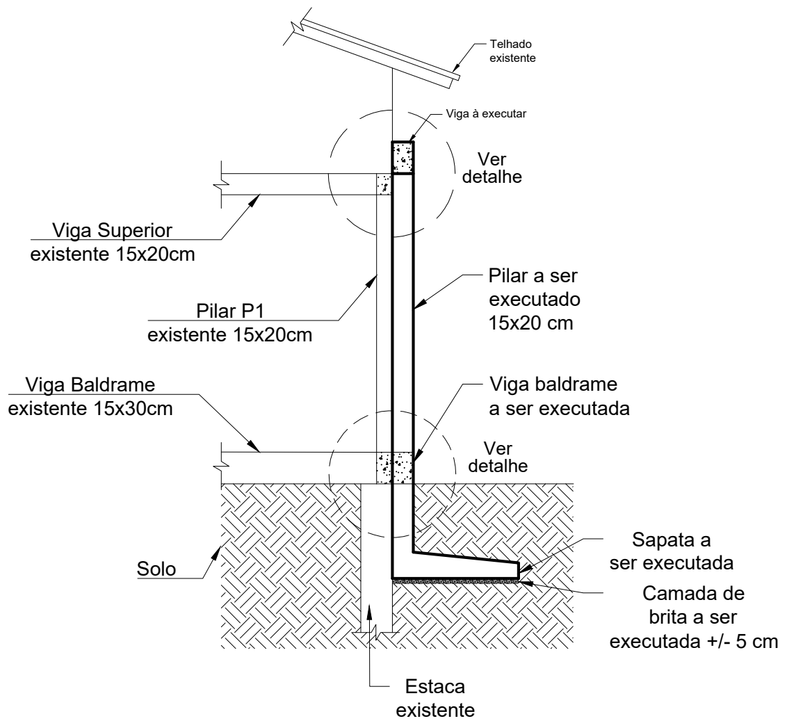
Corte esquemático Esc. 1/50
